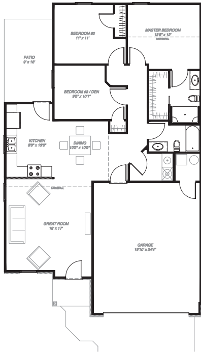
OPTIONAL 3-BEDROOM PLAN
